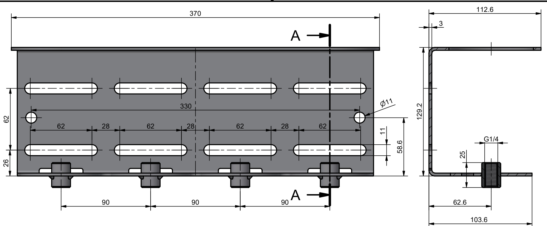
A-A ( 1 : 2 )
