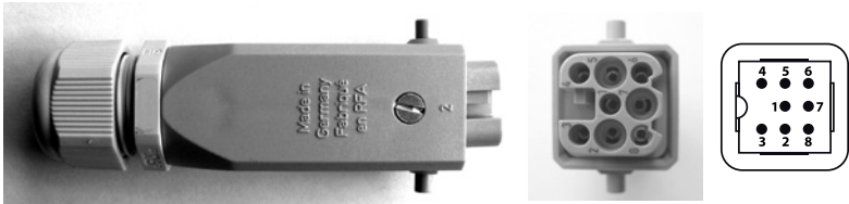
Abb. 10-2: Steckverbindung B (8-polig) für Anschluss der Steuerung
