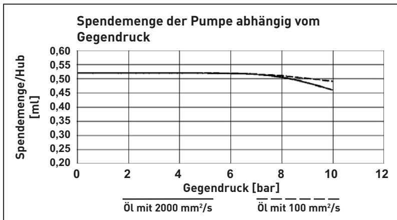
Abb. 9-1 Spendemenge der Pumpe abhängig vom Gegendruck
